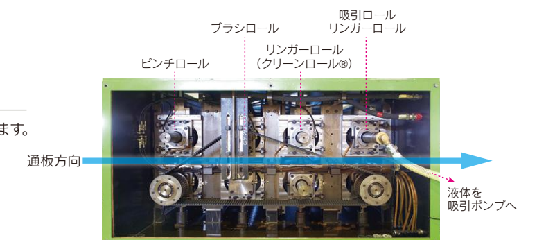
自動車用吸引ユニット付鋼板洗浄試験機
